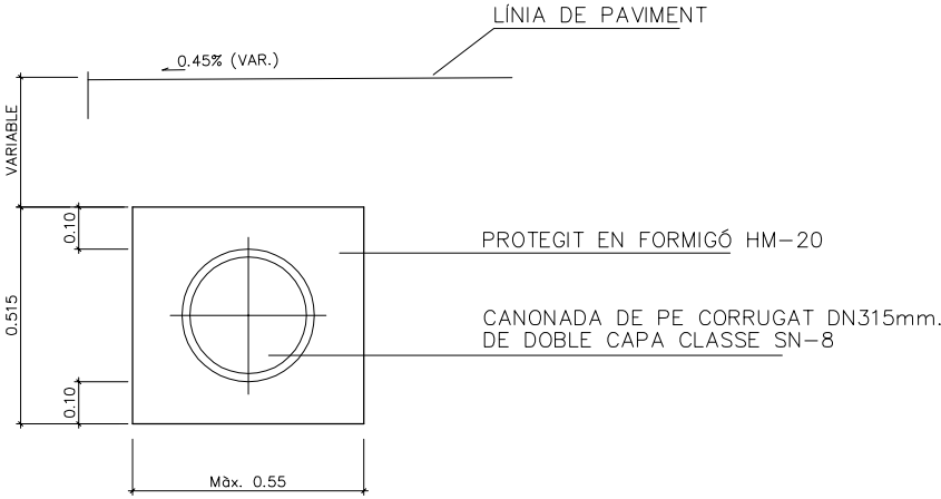
SECCIÓ K-K PROTECCIÓ DE CANONADA E: 1 / 20
