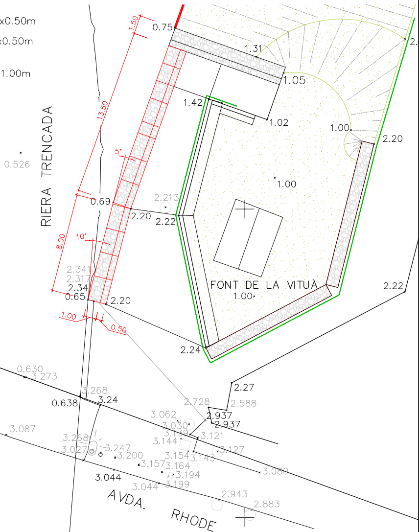
PLANTA GENERAL E: 1/300
