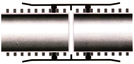
UNIÓ MITJANCANT MANIGUET H/H
