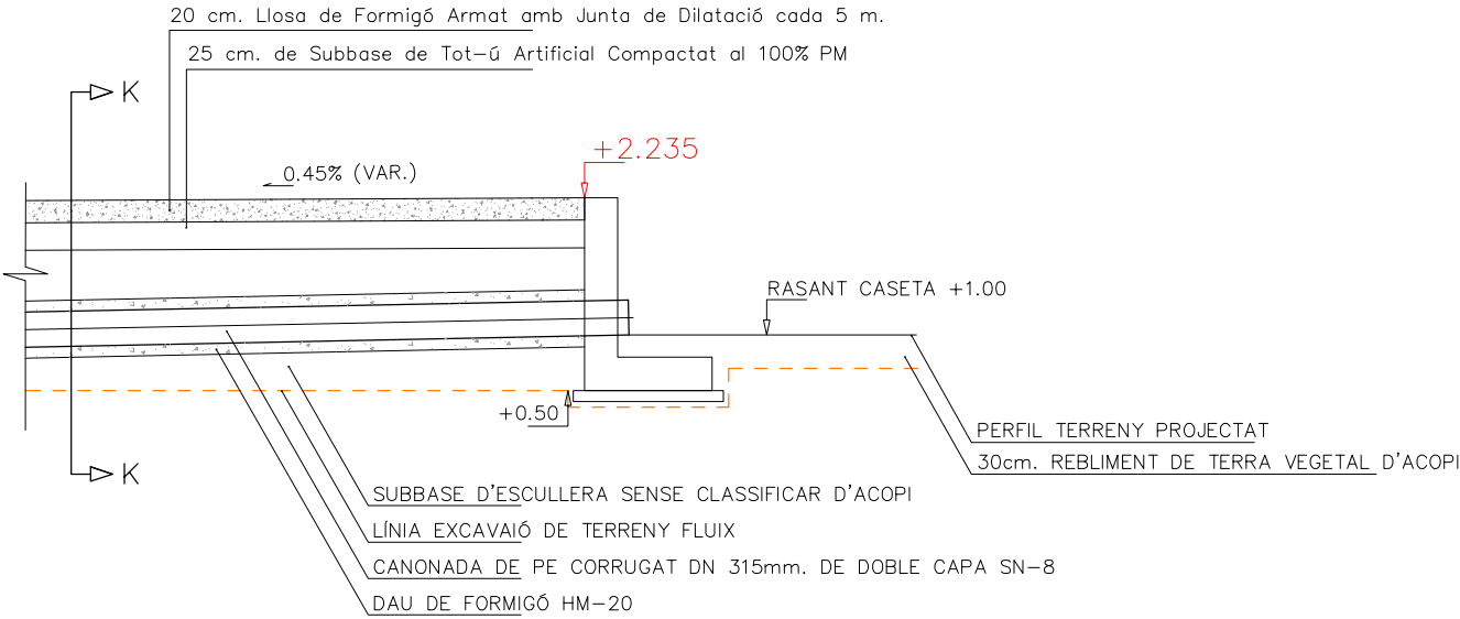
DETALL-SECCIÓ J-J E: 1/75
