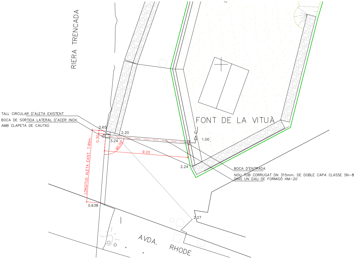
PLANTA GENERAL E: 1/200
